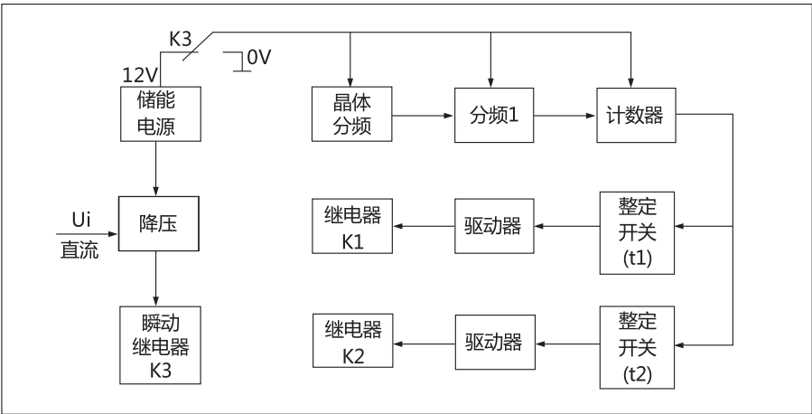
图1 继电器原理框图
